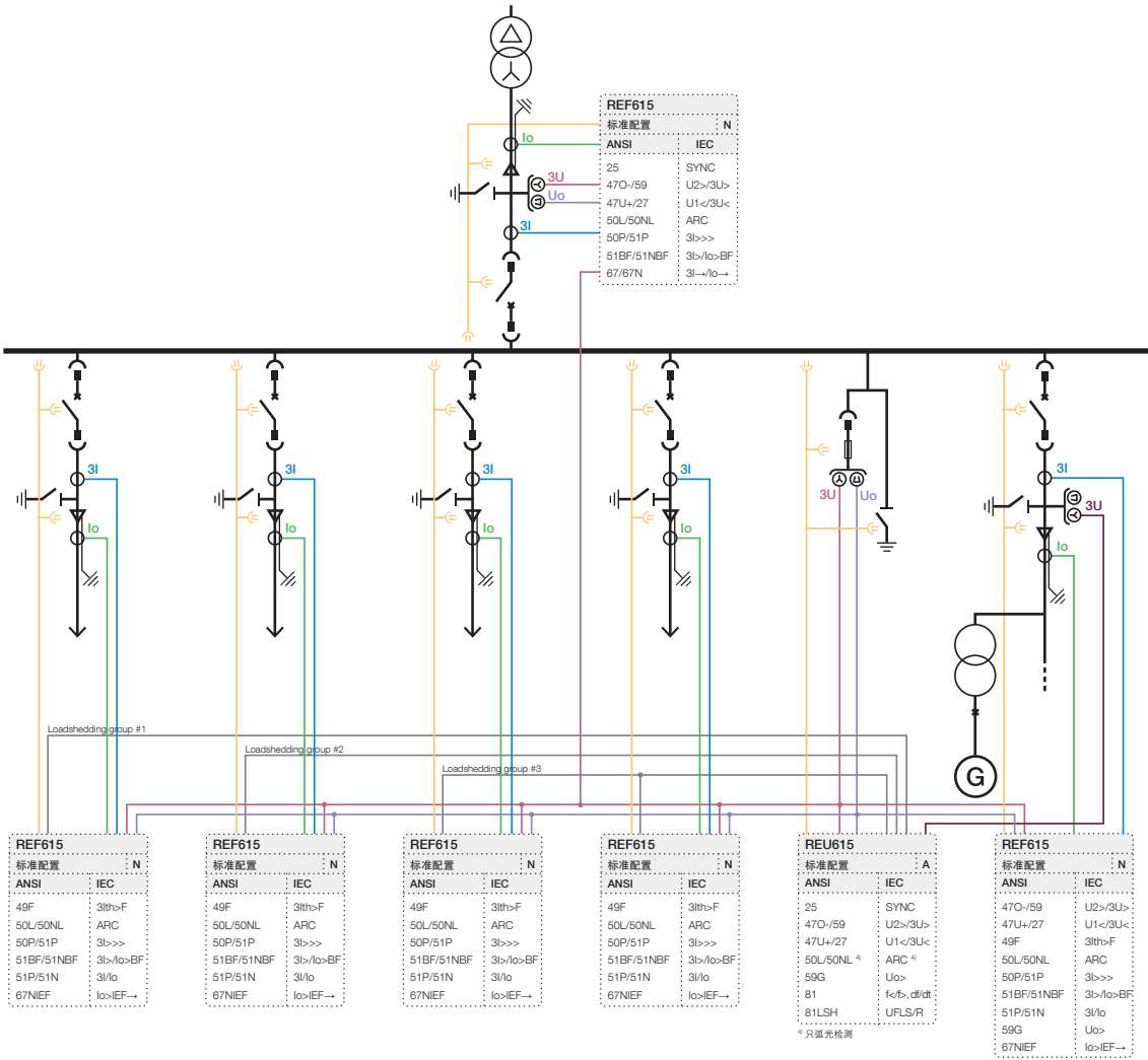
图3：采用REU615标准配置A实现对母线的保护和监视
