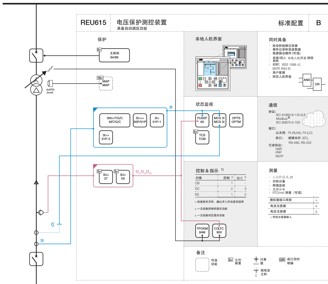
图2: 标准配置B的功能总览
