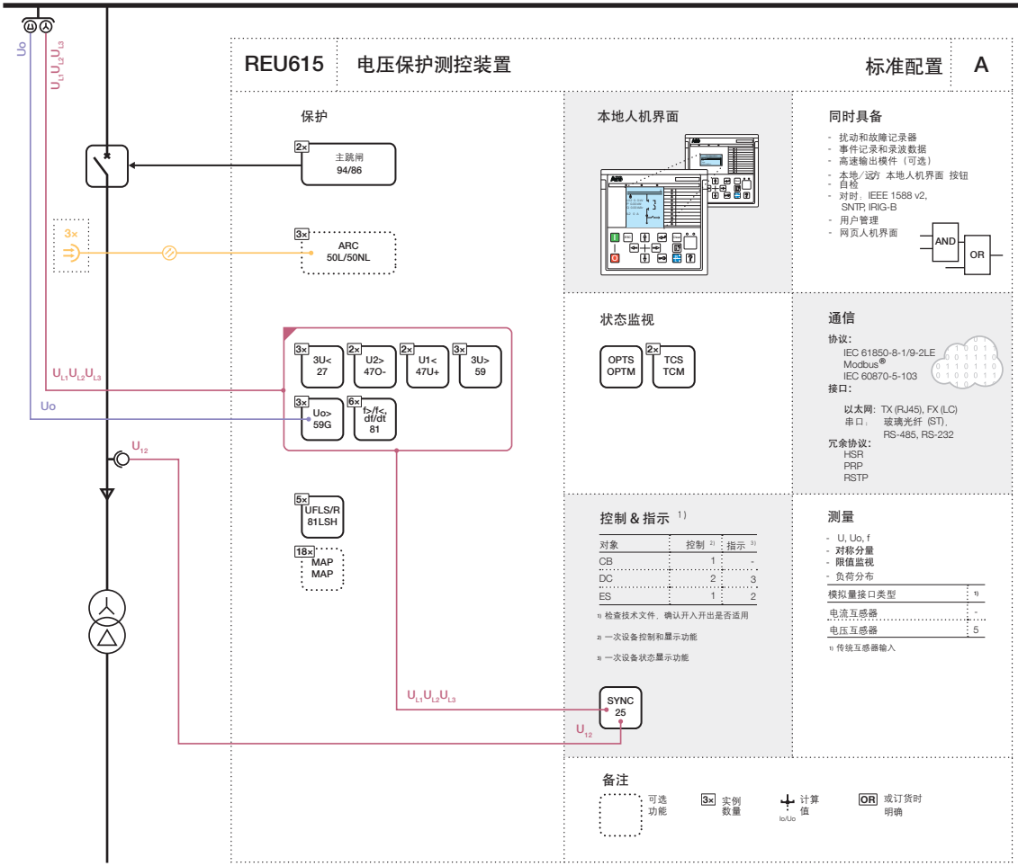
图1：标准配置A的功能总览
