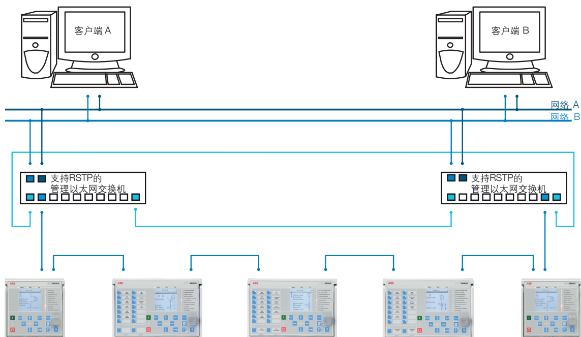
图9：自愈环网解决方案
