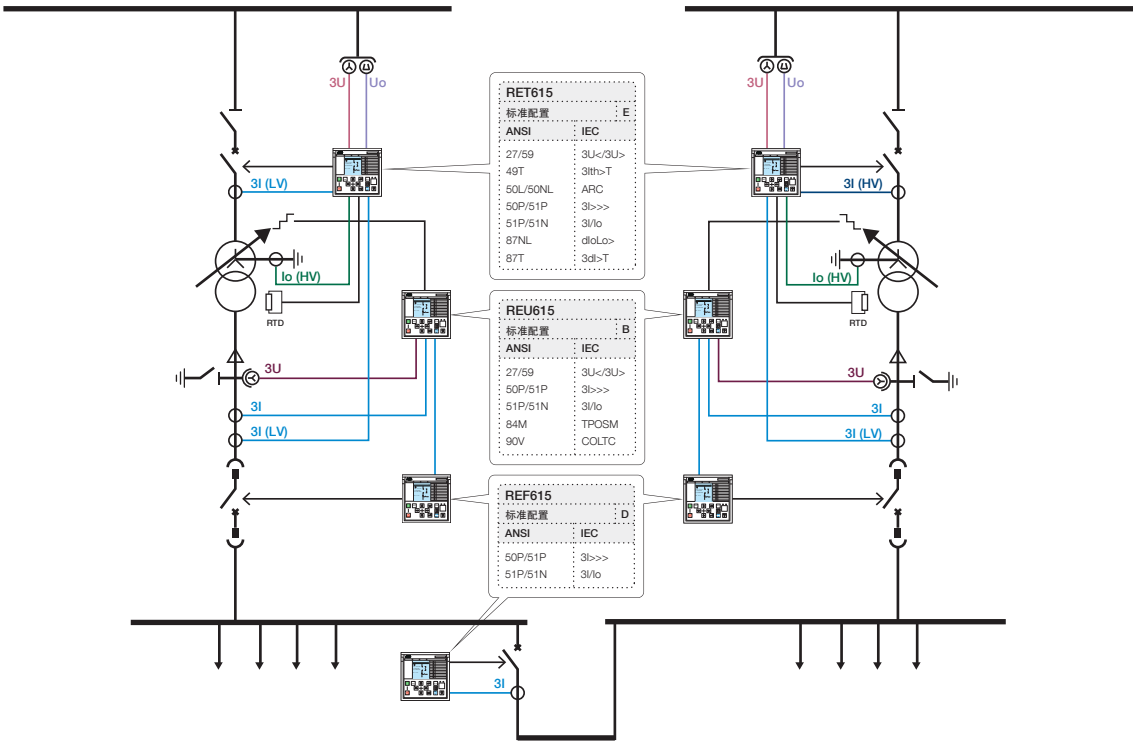
图4：采用具备标准配置B的REU615实现对分接开关的控制和电源变压器的热过负荷保护
