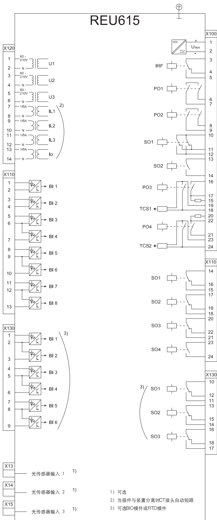
图16: 标准配置B的 接线图
