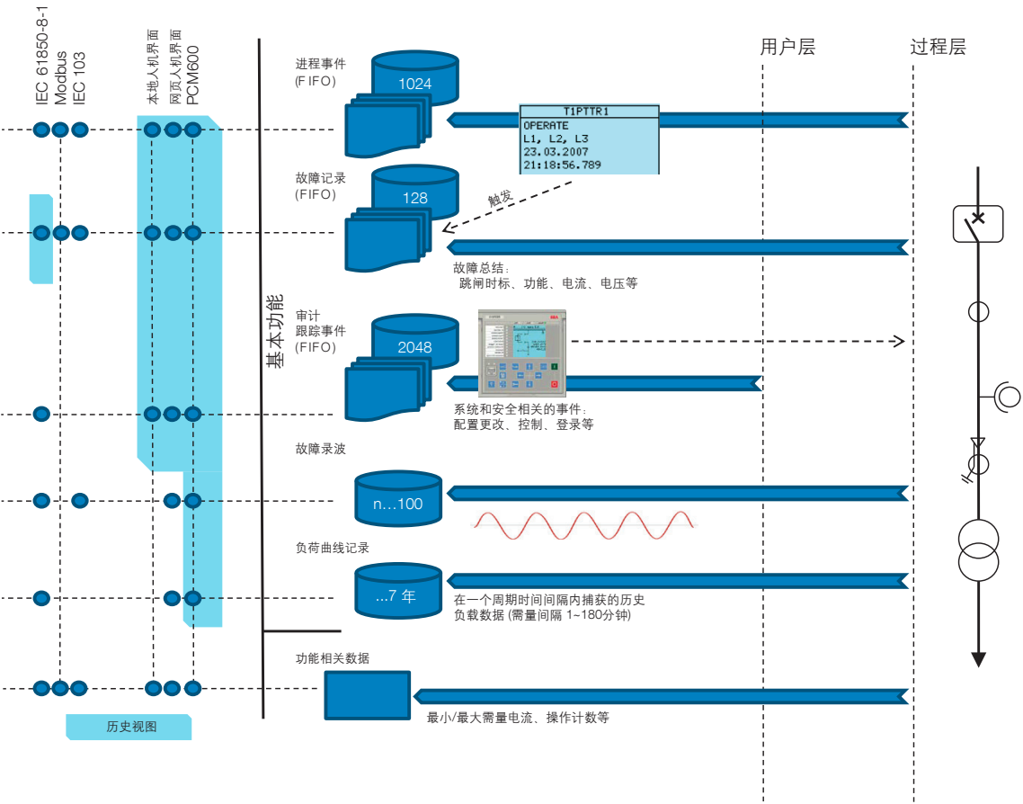
图6：录波和事件功能概述
