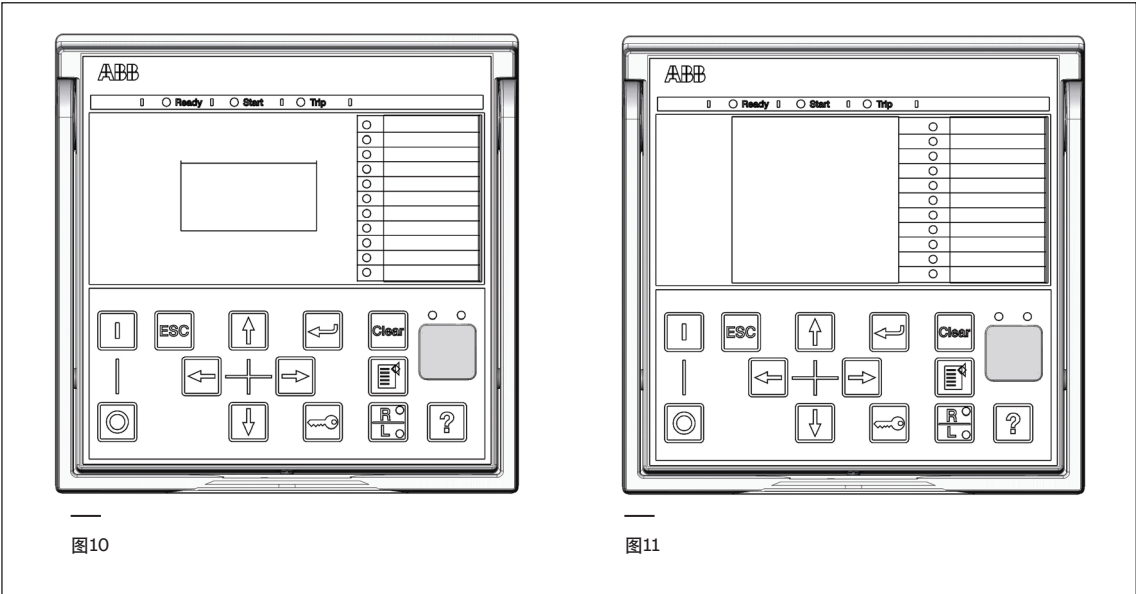
图10：小屏幕显示屏
