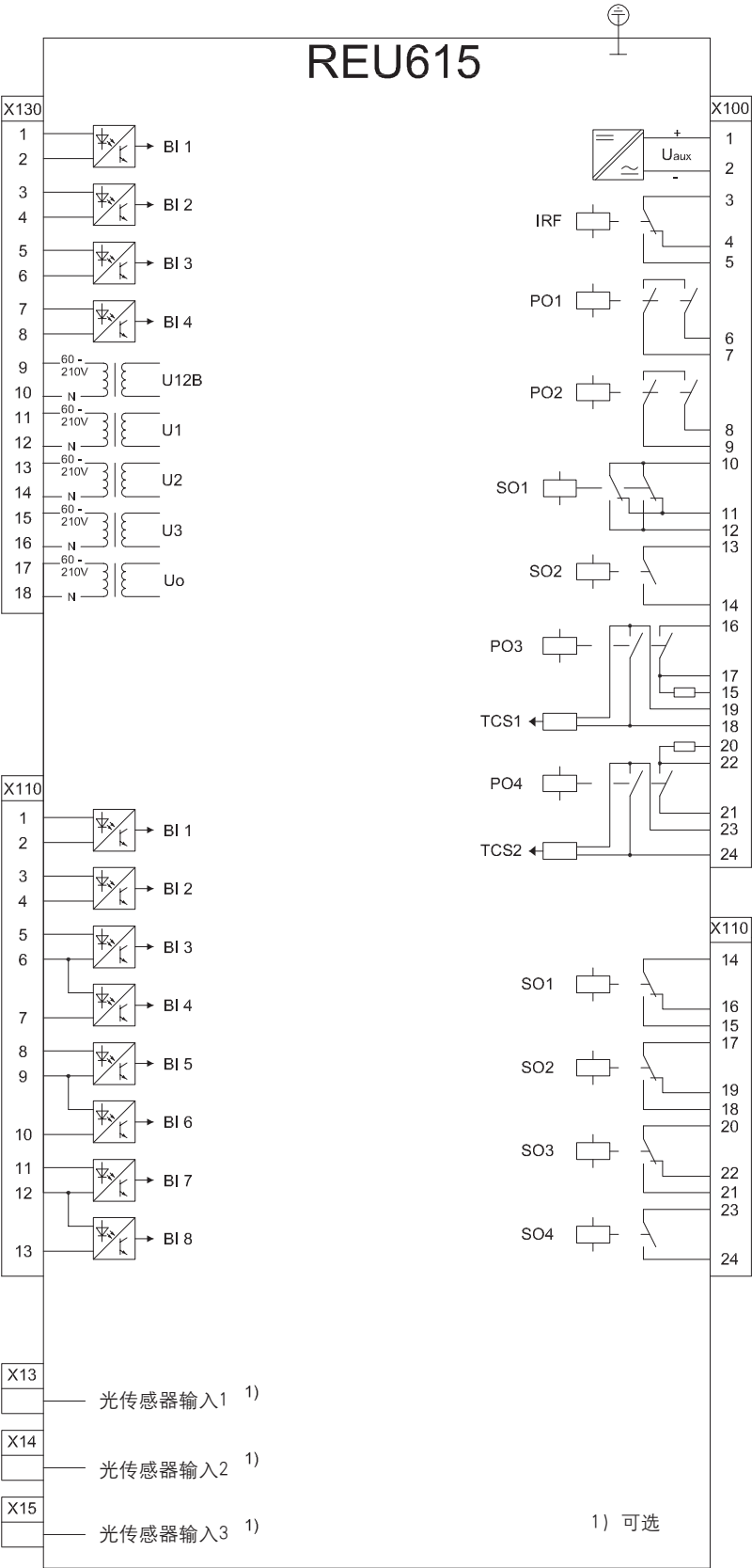
图15：标准配置A的接线图
