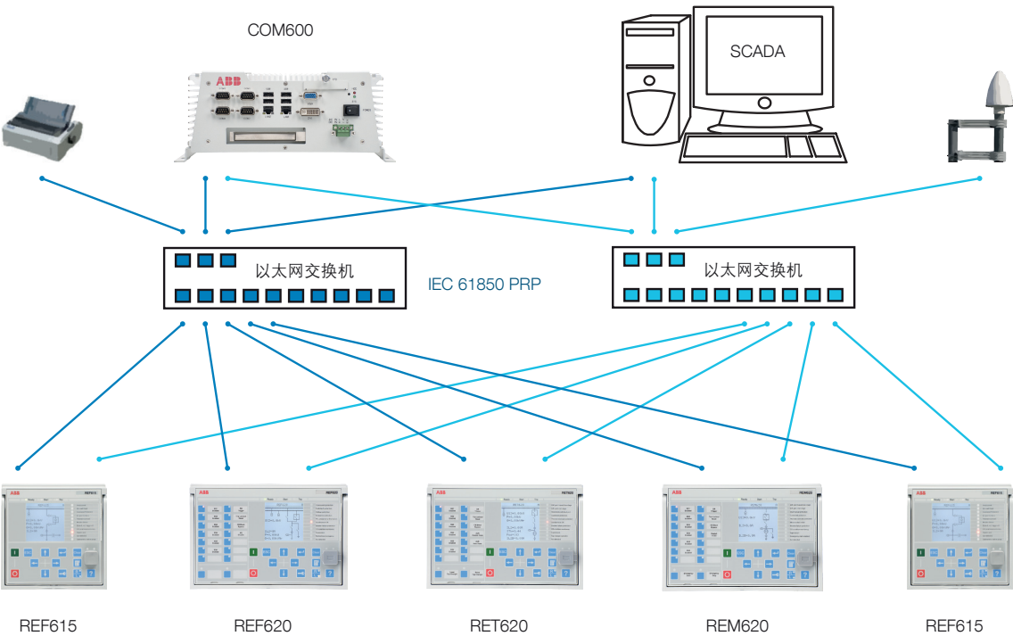
图7：平行冗余协议 (PRP)解决方案
