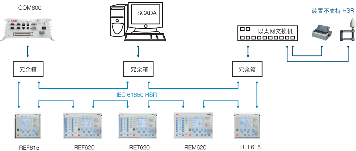
图8：高可用性无缝冗余协议(HSR)解决方案
