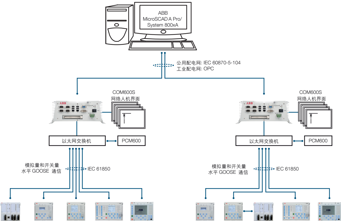
图5：ABB电力系统使用Relion®继电器，COM600和MicroSCADA Pro / System 800xA样例
